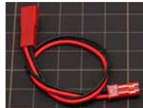
0019-09 延長コネクタ (BEC-BEC) JST-BECコネクタの延長に使用。
